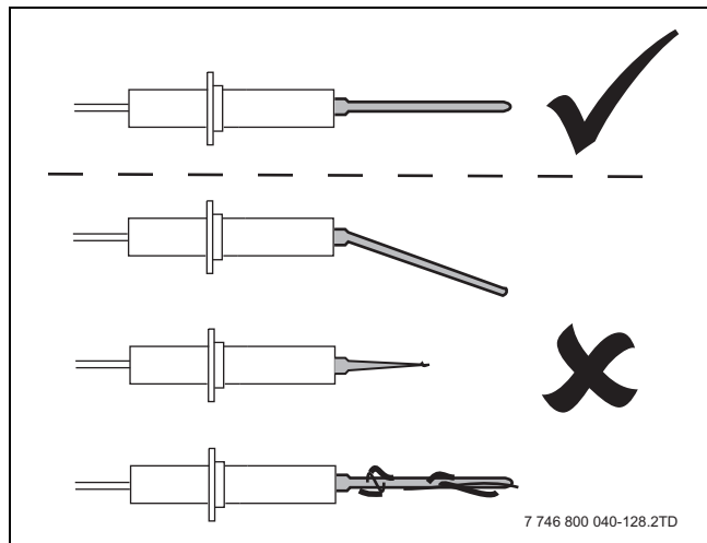
Рис. 63 Проверка контрольного электрода
