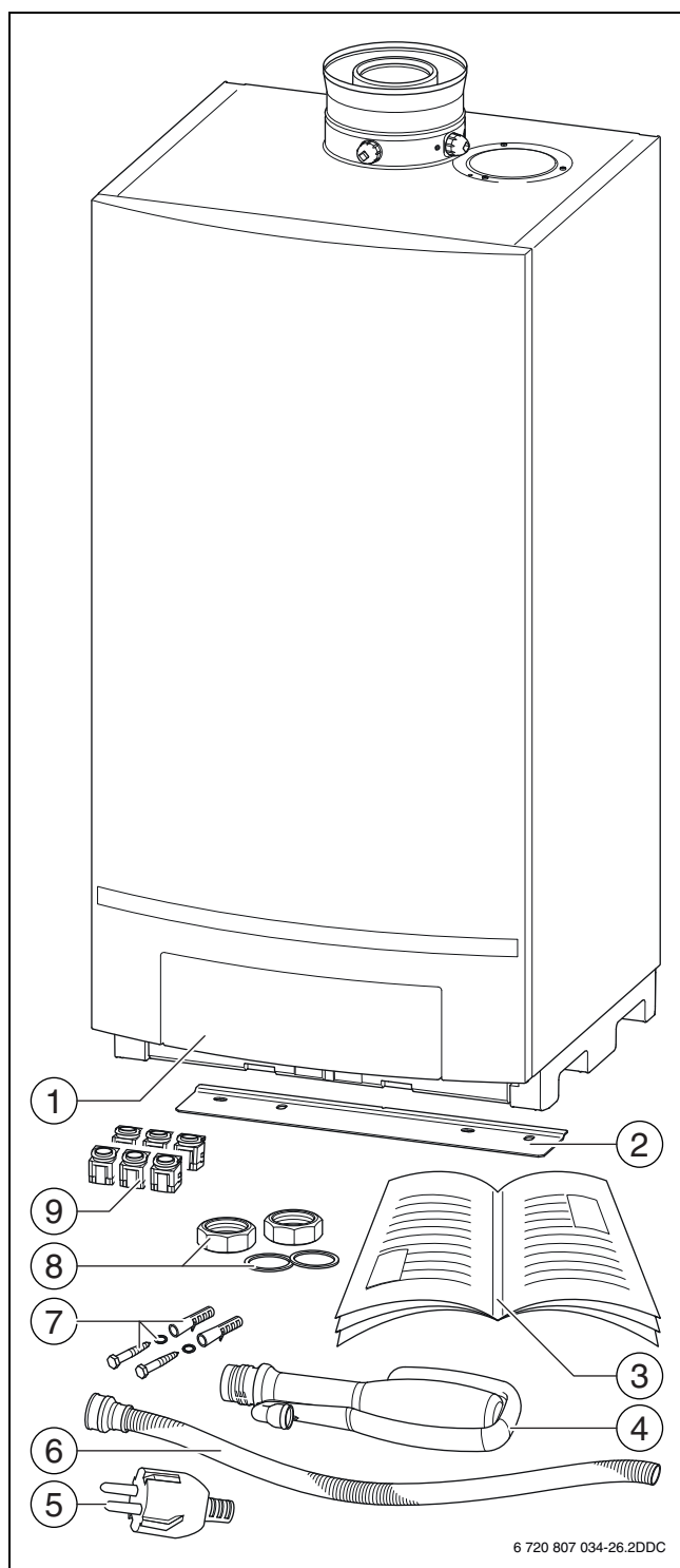
Рис. 1 Комплект поставки
