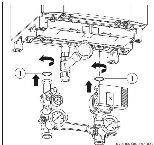
Рис. 14 Монтаж группы подключения
