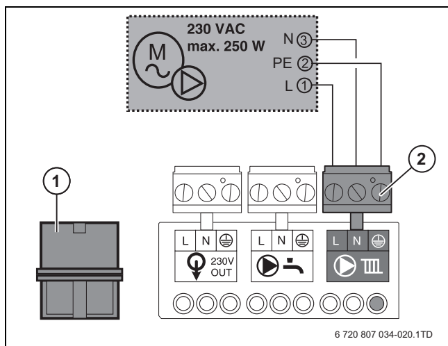
Рис. 43 Подключение насоса
