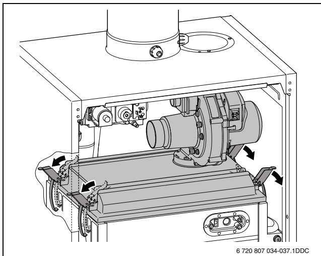
Рис. 58 Раскрытие защёлок
