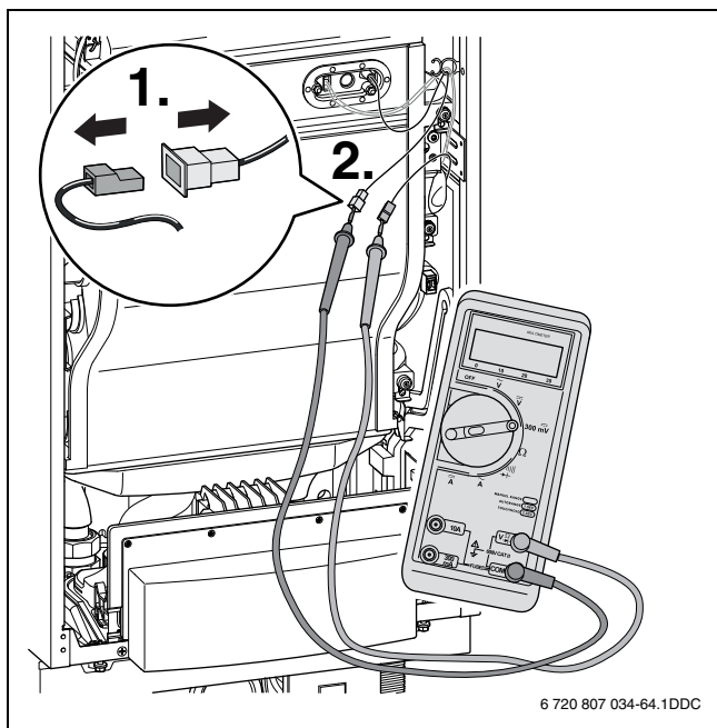
Рис. 53 Подключение мультиметра
