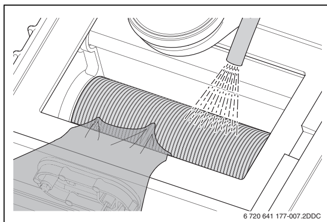
Рис. 62 Чистка теплообменника
