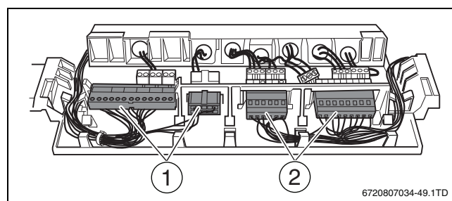
Рис. 27 Клеммные колодки
