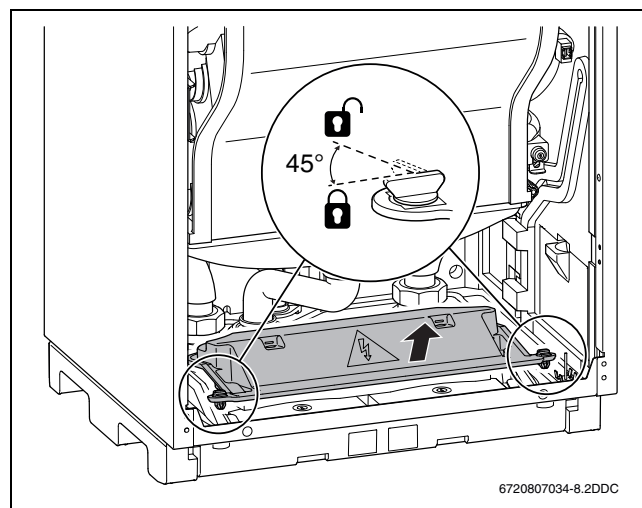
Рис. 26 Снятие крышки
