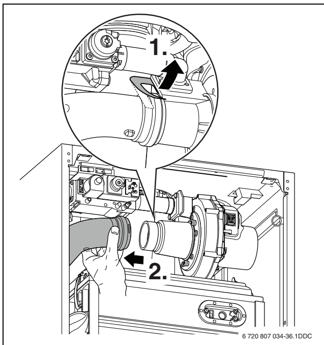
Рис. 57 Отсоединение воздухозаборной трубы (выноски: тип 70)
